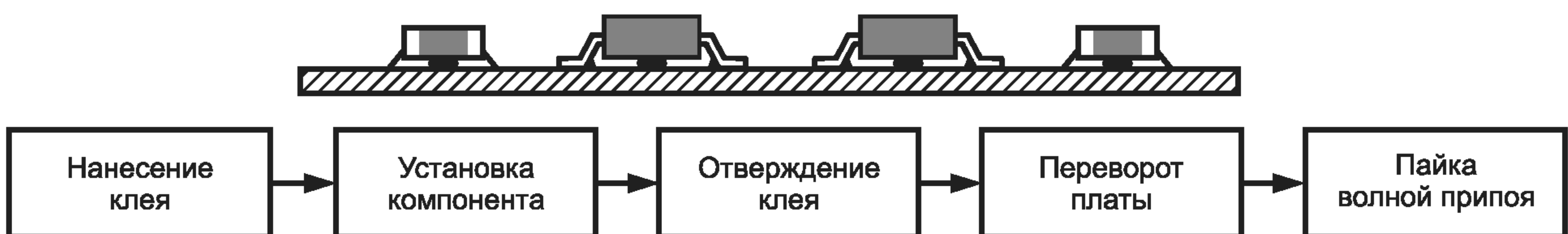
Рисунок 2 — Односторонний печатный узел. Пайка только погружением
