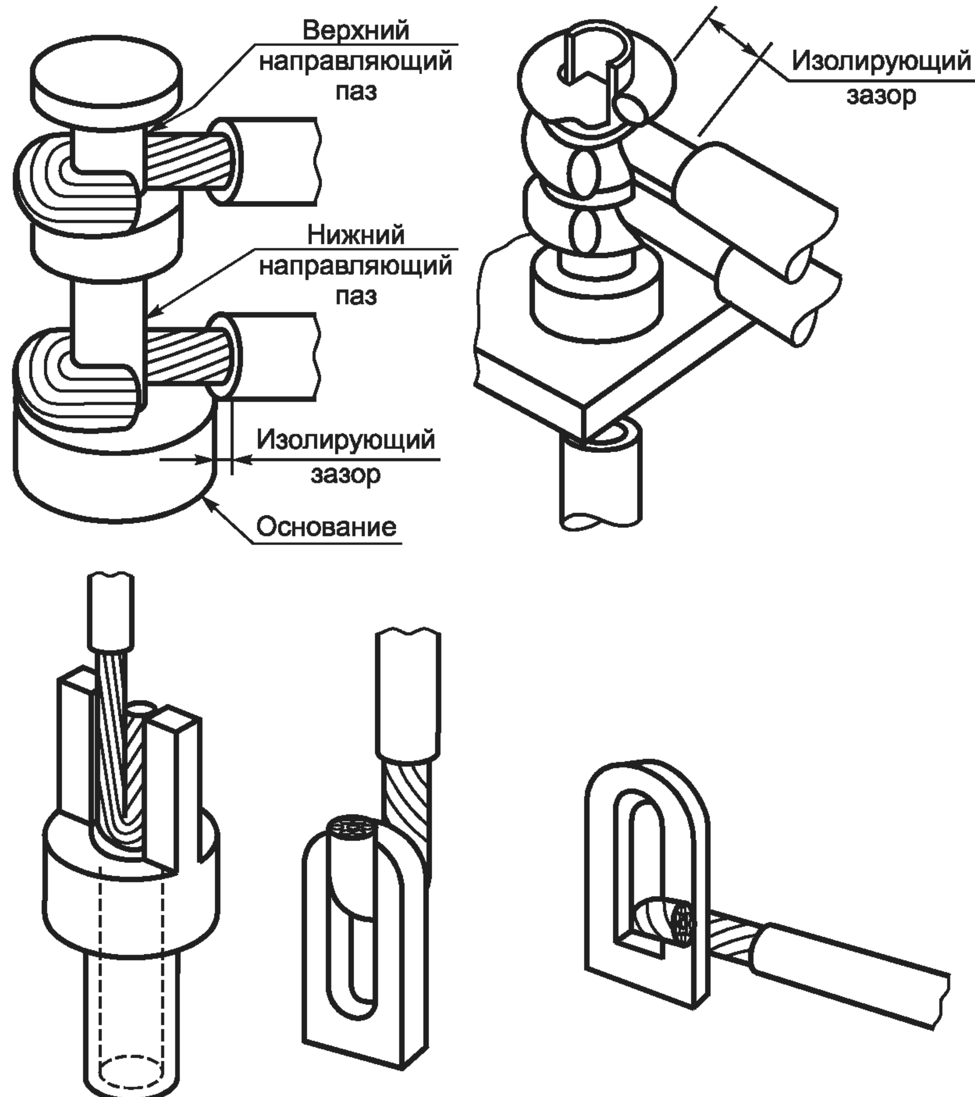
Рисунок 15 — Виды закрепления провода
