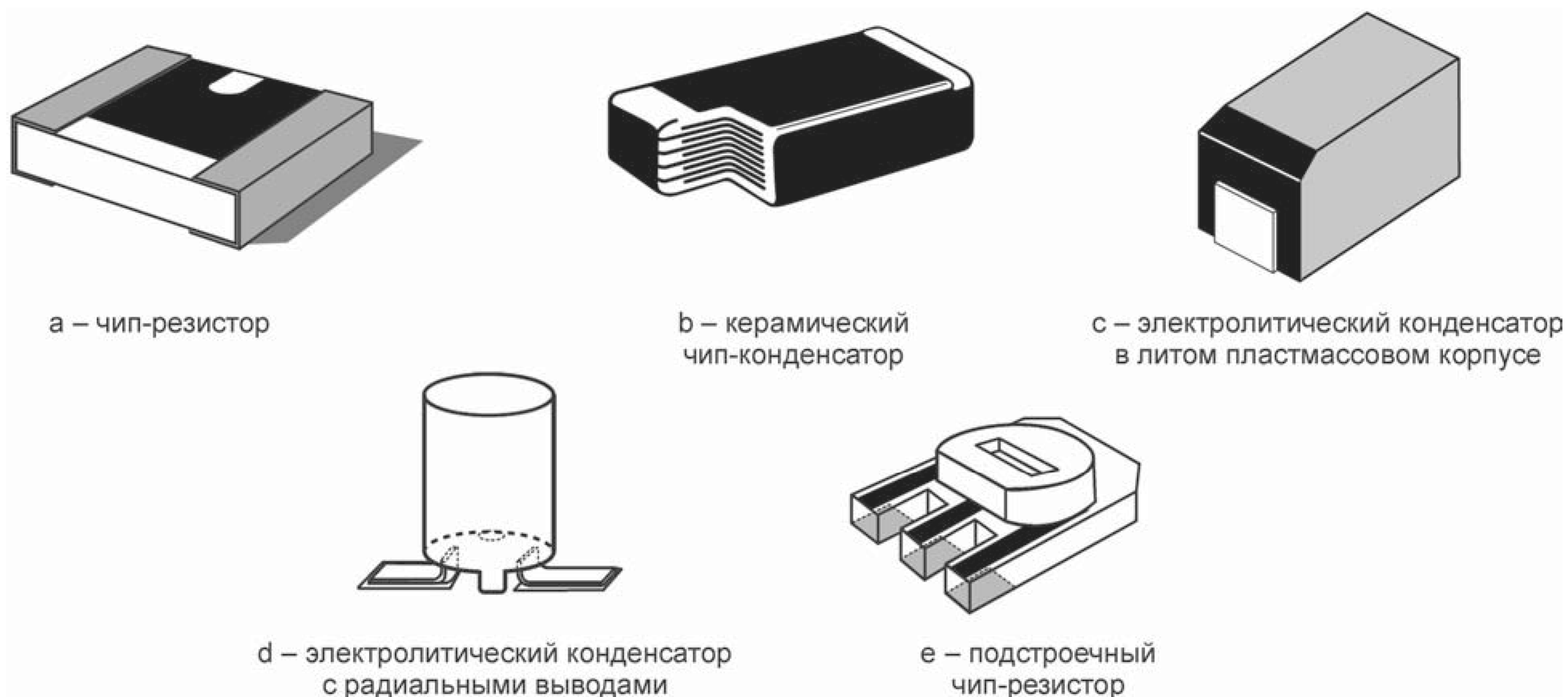
Рисунок 6 — Типовые конструкции корпусов пассивных и активных компонентов поверхностного монтажа
