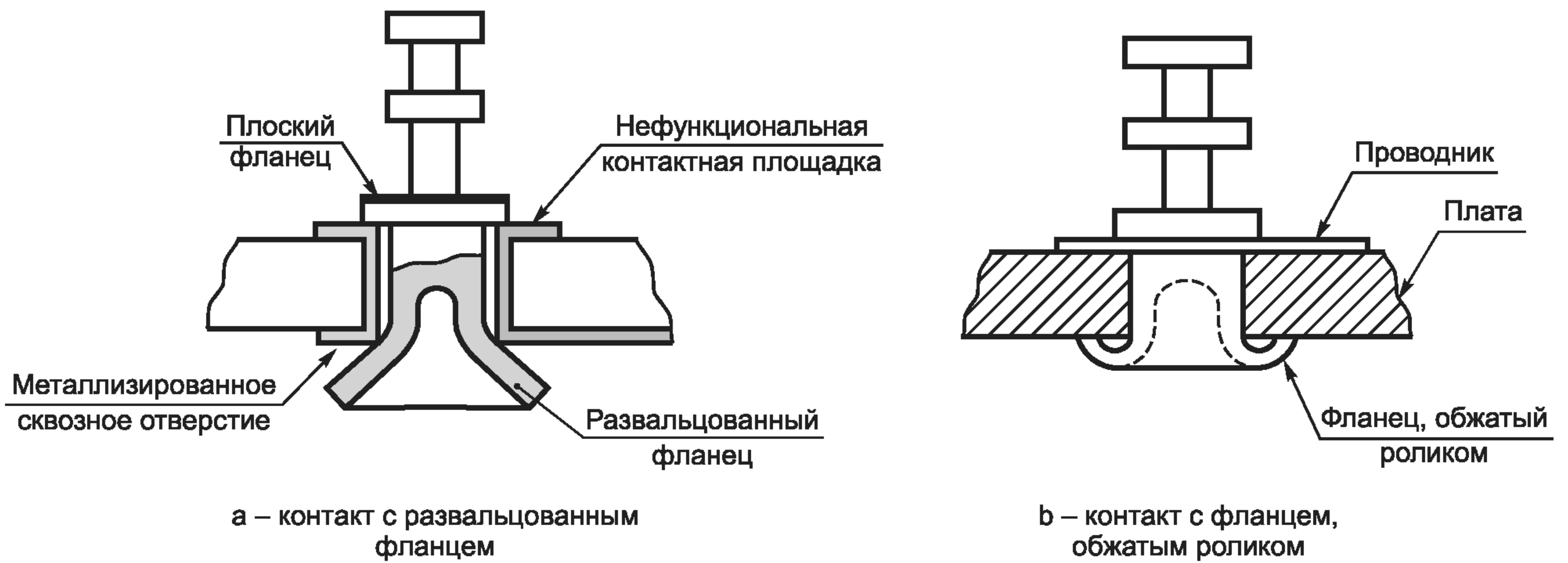
Рисунок 14 — Примеры закрепления контактов
