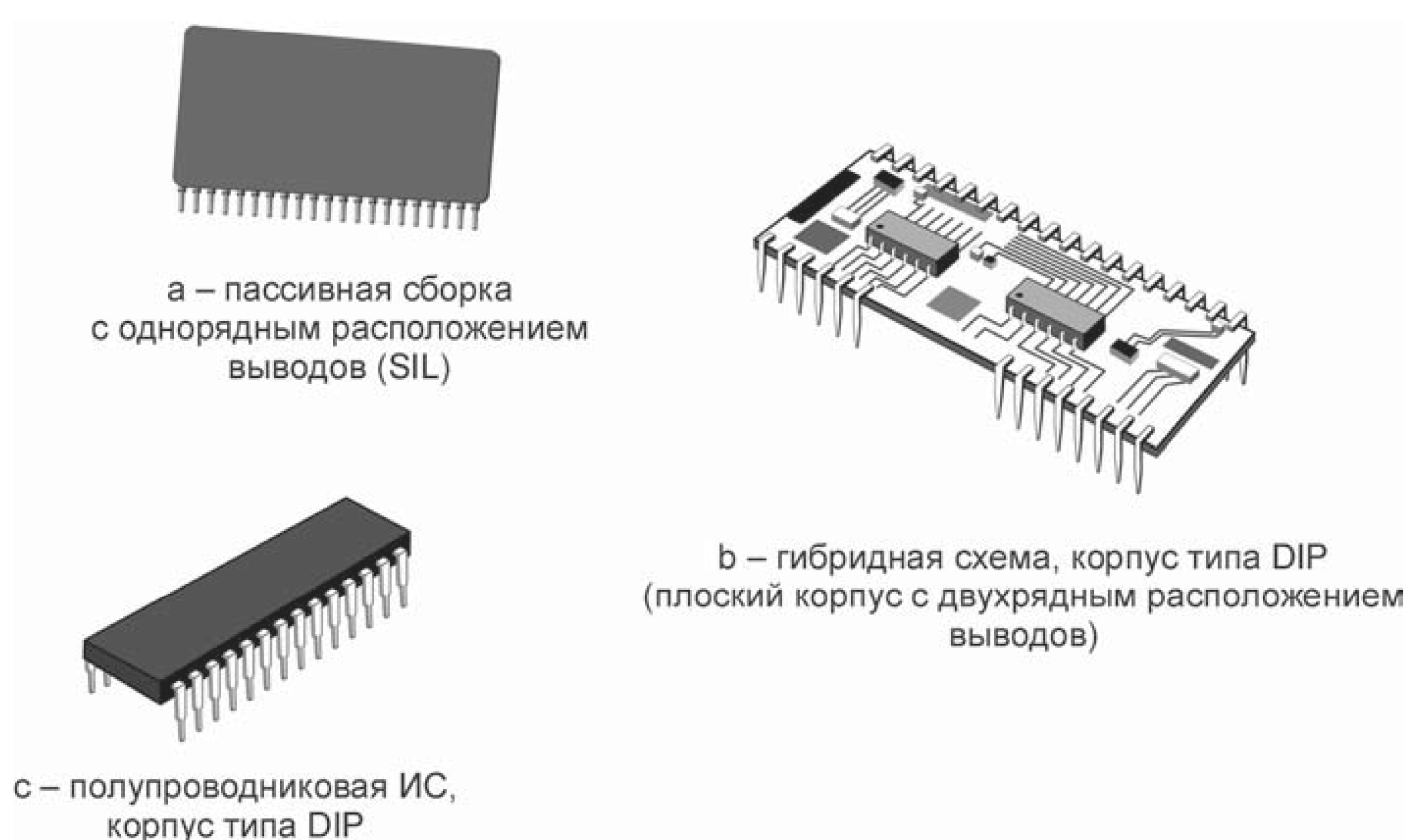
Рисунок 12 — Типовые конструктивные исполнения многовыводных корпусов ИС
