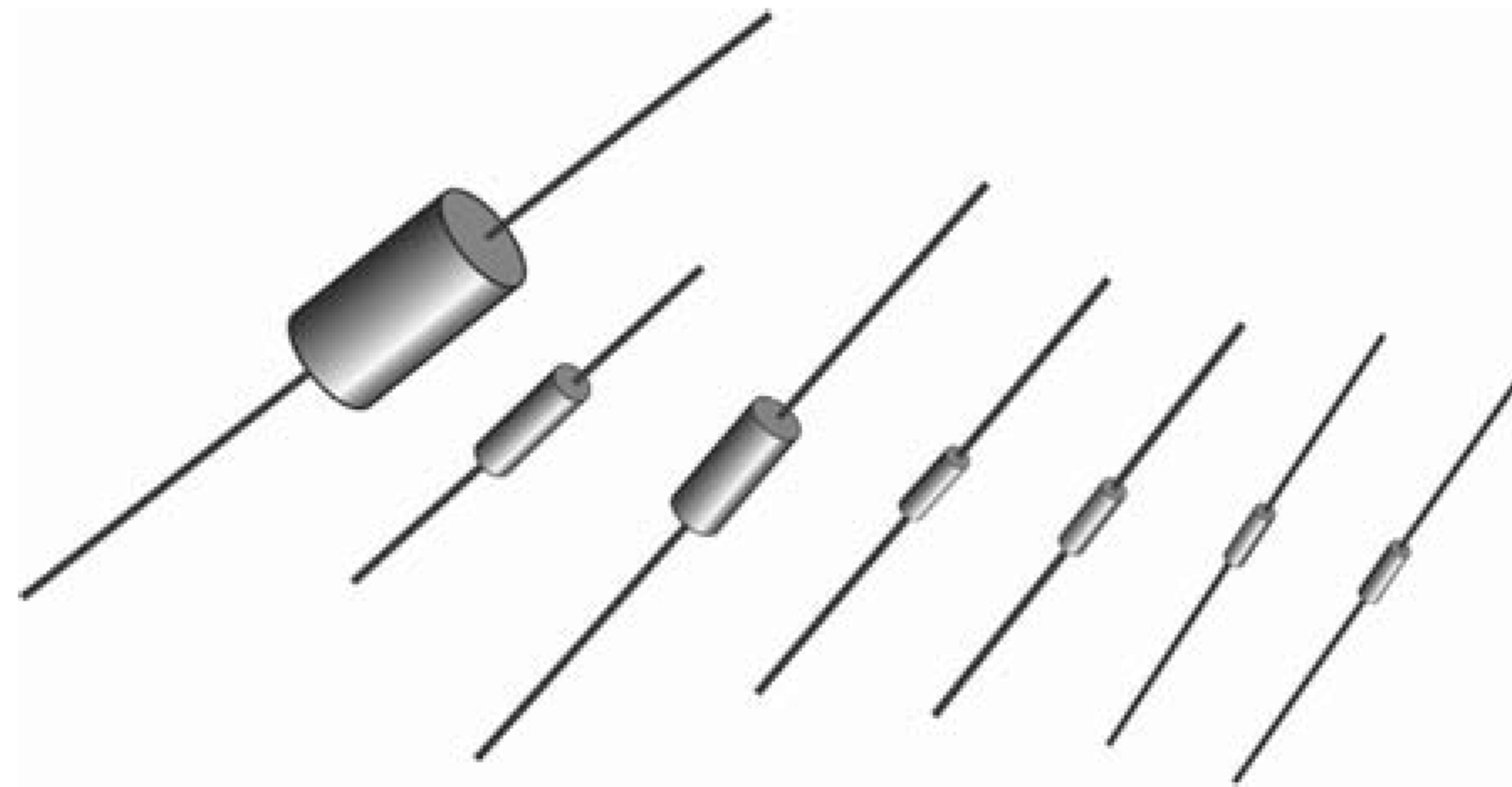
Рисунок 8 — Типовые компоненты с коаксиальными выводами
