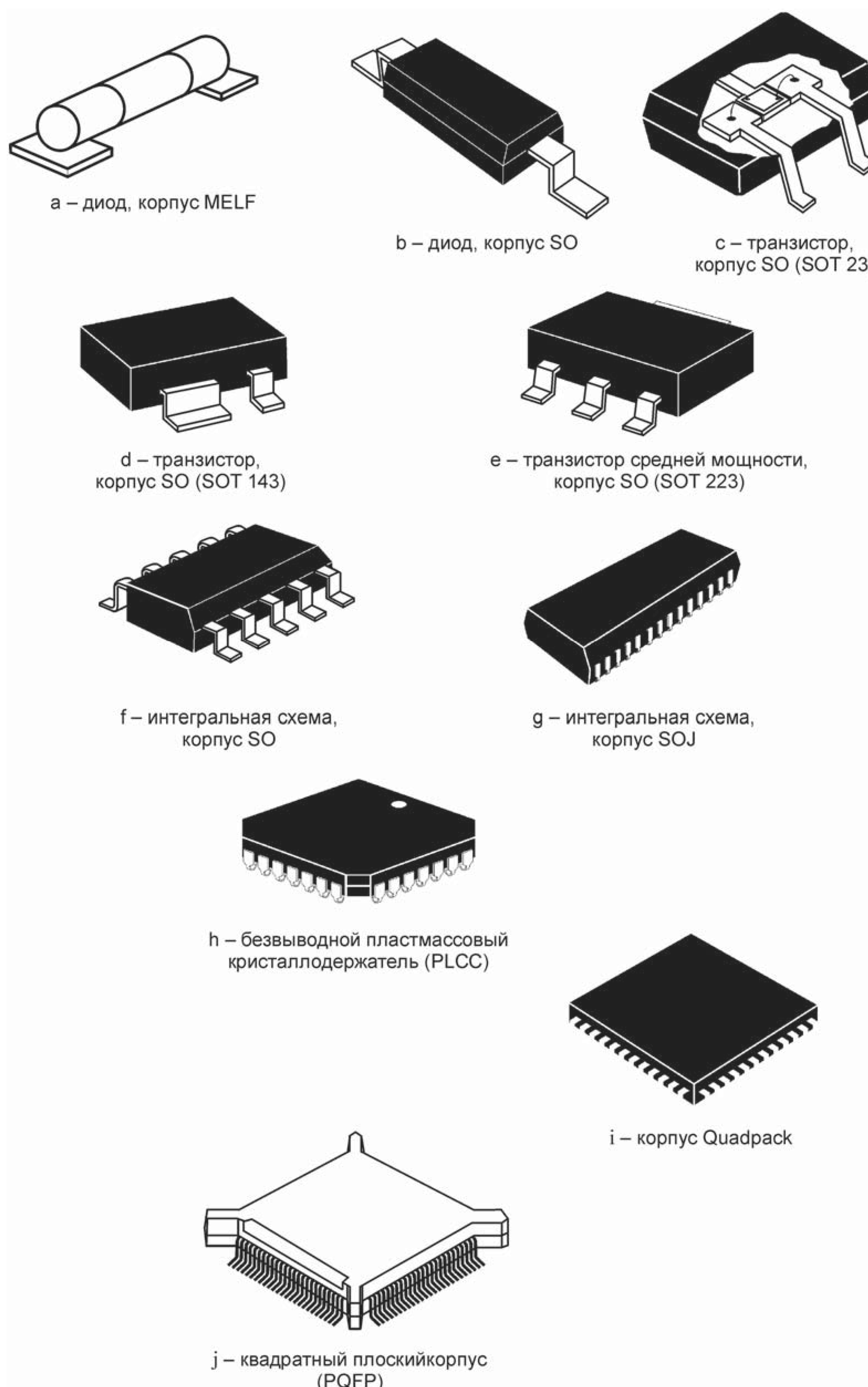
Рисунок 7 — Типовые конструкции корпусов полупроводниковых компонентов поверхностного монтажа
