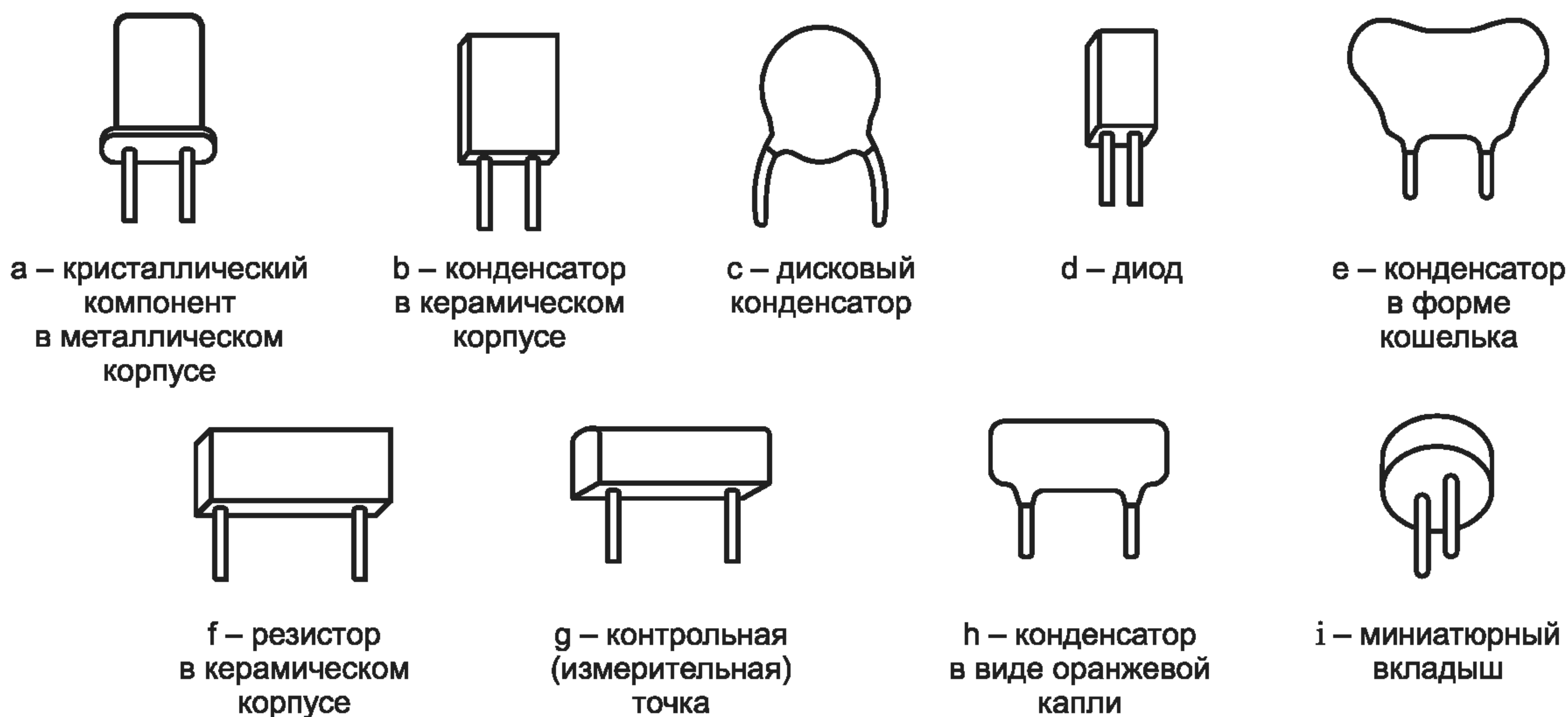
Рисунок 9 — Типовые компоненты с двумя радиальными выводами
